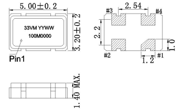
图1.外型说明
