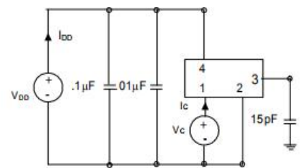
图2.典型输出测试条件
