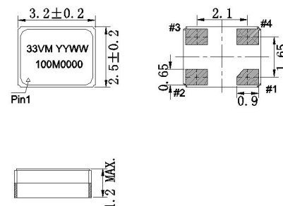
图1.外型说明
